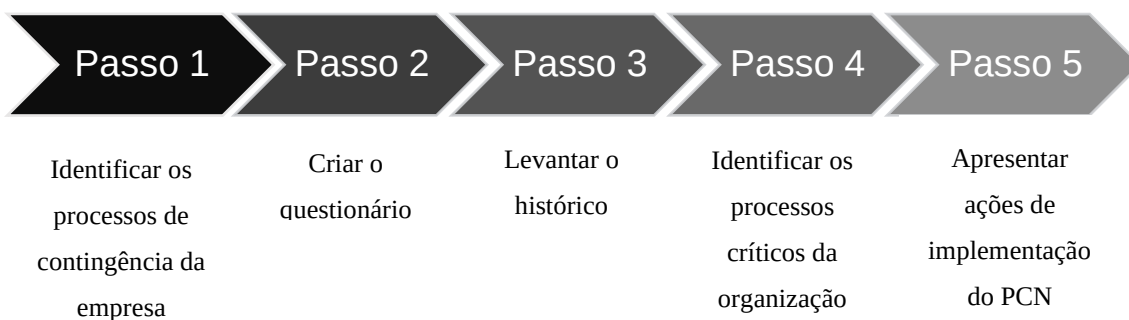
Figura 3 - Procedimentos Metodológicos
