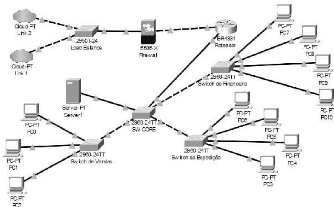
Figura 6: Sugestão do Diagrama de Rede da Empresa
